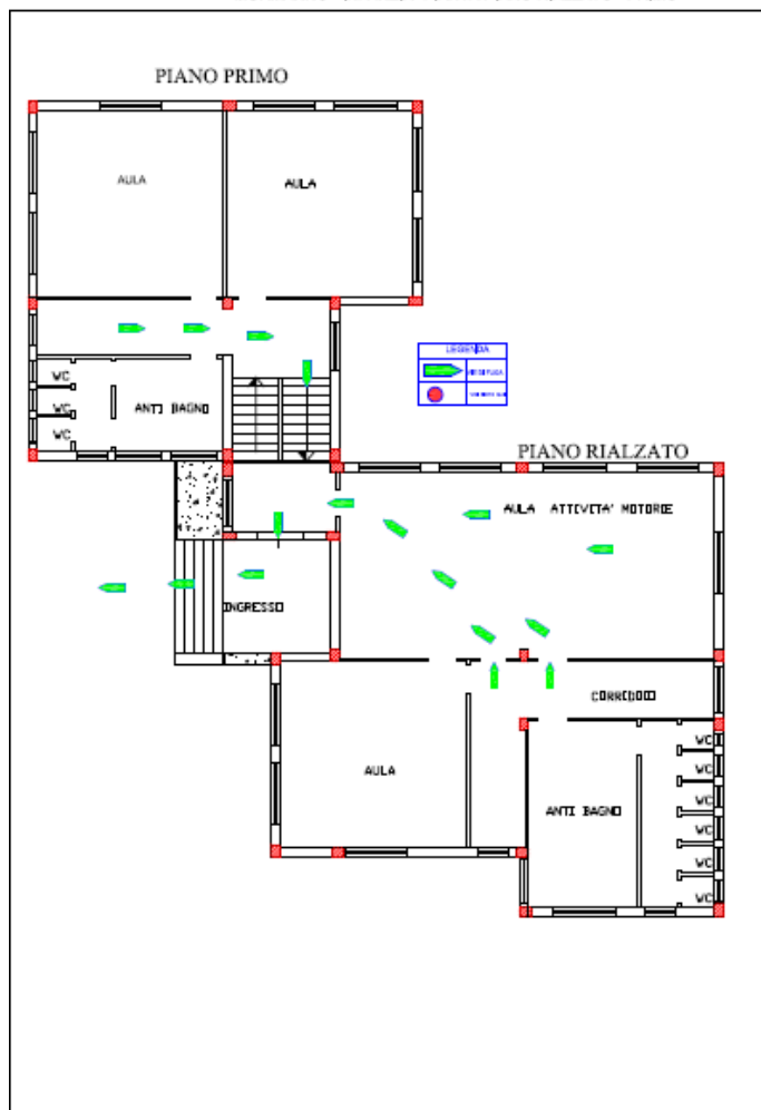
MORMANNO - INFANZIA- PIANTA PIANO RIALZATO - PRIMO
